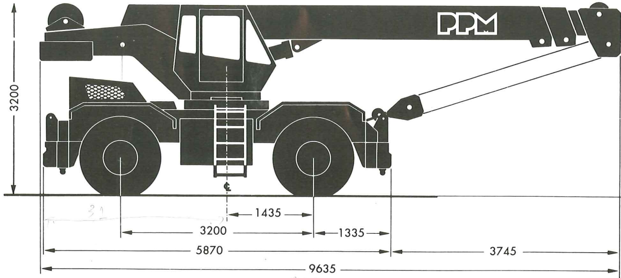
Dimensions en mm
