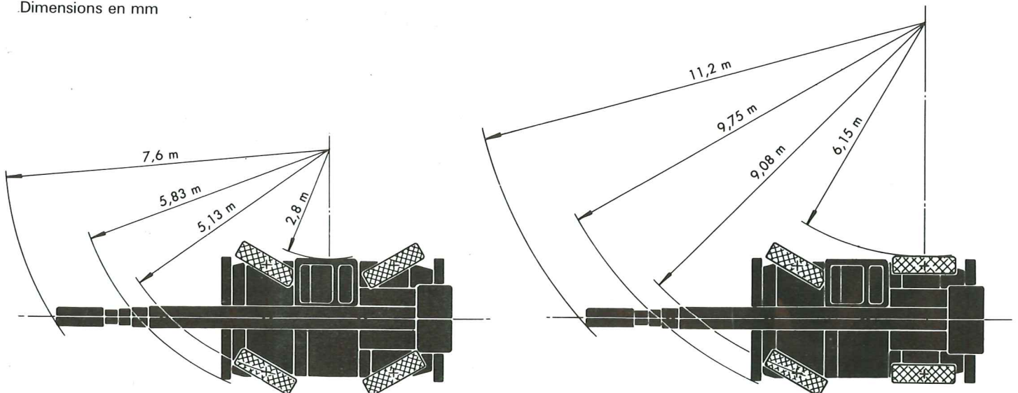
Dimensions en mm
